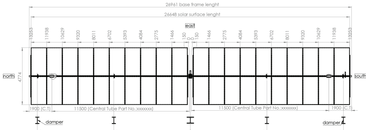
DEGER S100-AG-DR mit Rammfundament (1)
